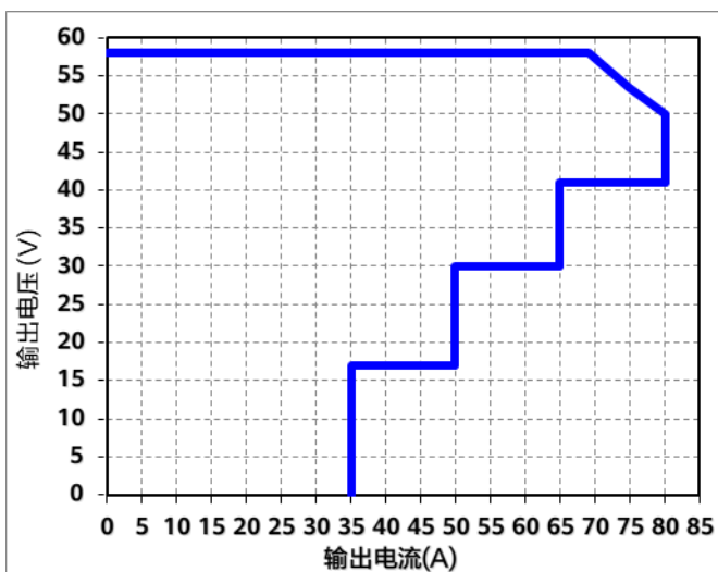
图2 输出效率曲线 (230V AC, 25°C)
